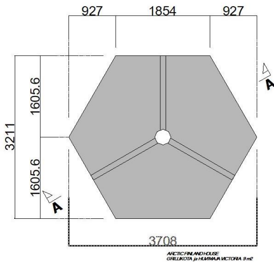
Grundriss der Fundamente
